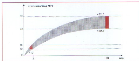
a cement szilárdulása az idő függvényében
